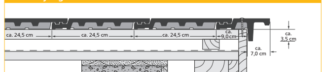
Halv høyre gavlkant *
