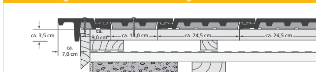
Halv venstre gavlkant med dobbeltfalset teglstein *
