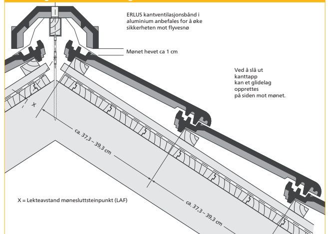
Mønetegl nr. 17 med flatetegl
