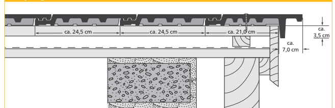
Høyre gavlkant*
