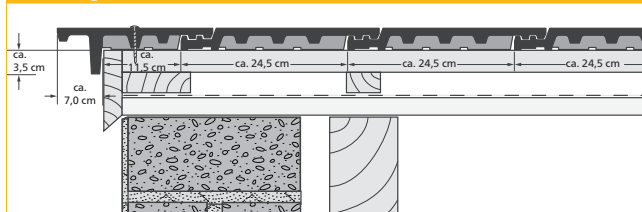
Venstre gavlkant*
