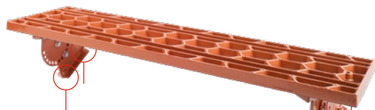
ALU-SYSTEM Rost 80 x 25 cm für Schornsteinfegerarbeiten nach EN 516
