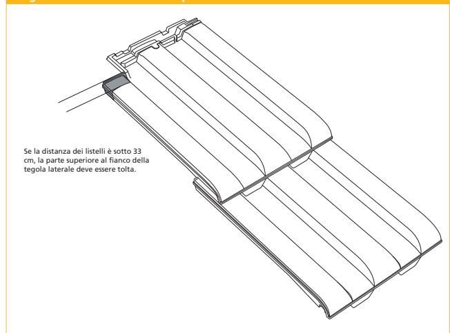
Tegola laterale – Istruzioni di posa
