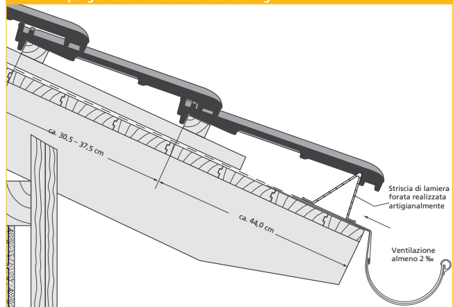
Gronda sporgente con sottotetto scarico in gronda
