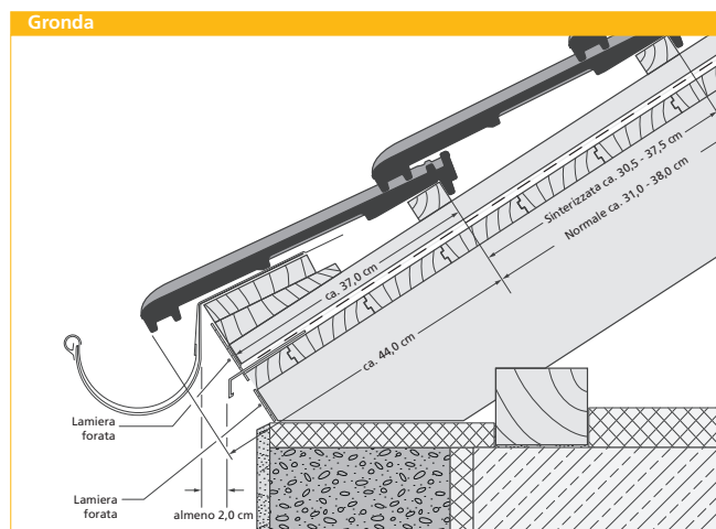
Gronda sporgente con sottotetto coibentato
