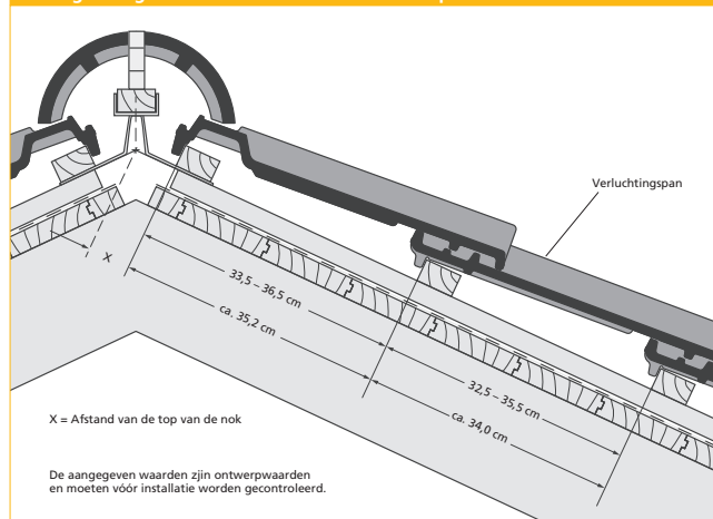
Droog verlegde vorst nr. 15 met vorstaansluitpan
